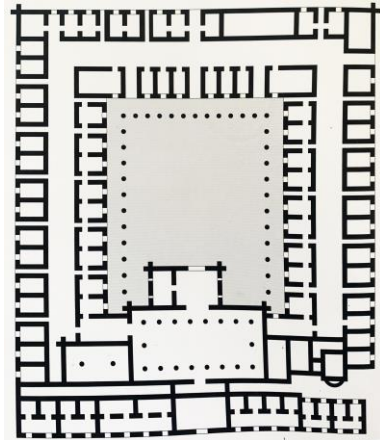
PLANTA VALETUDINARIUM DE ROMA
