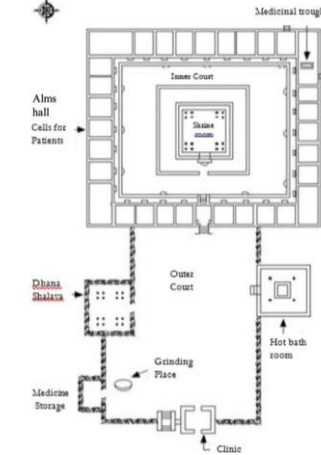
PLANTA HOSPITAL DE MIHINTALE
